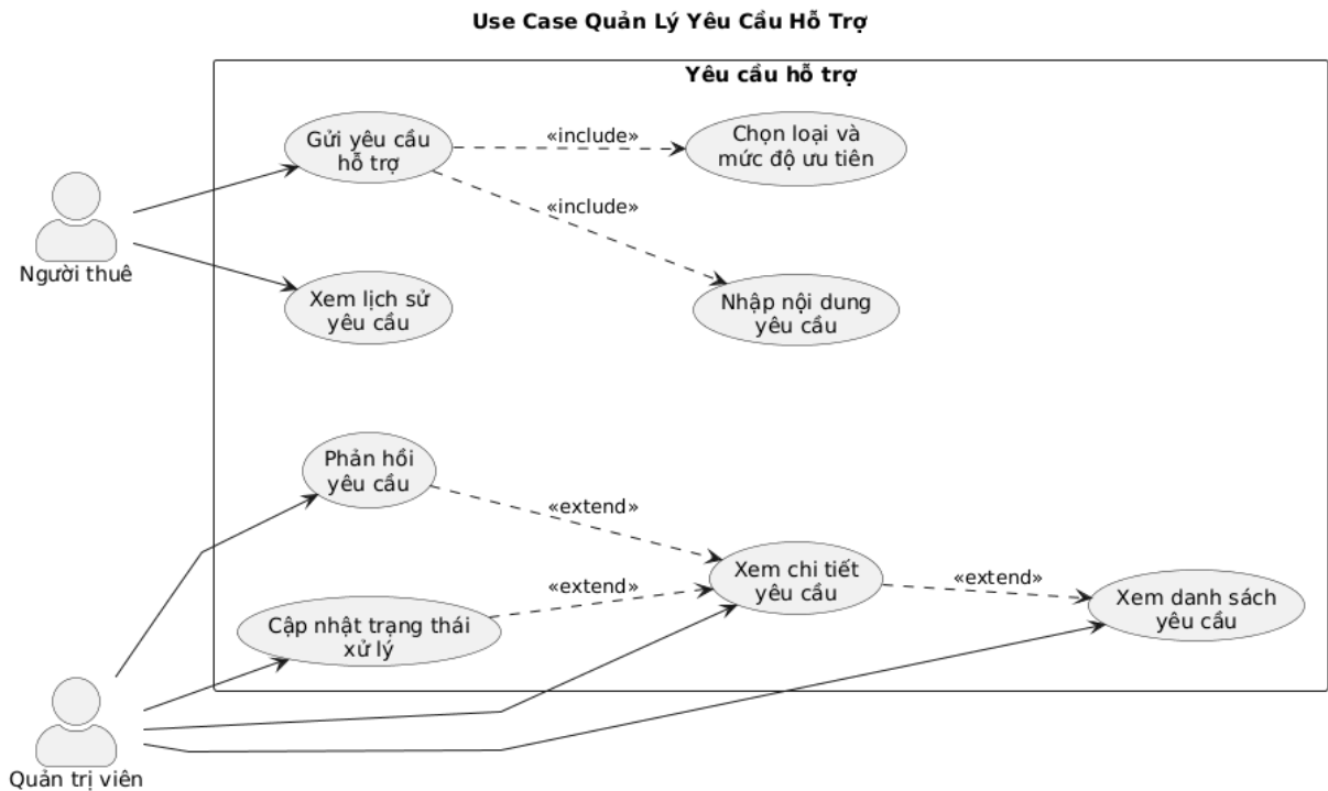
Hình 3.10 Sơ đồ Use case quản lý yêu cầu hỗ trợ
